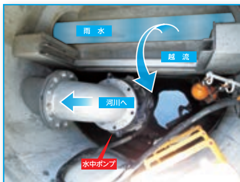
水中ポンプ据付状況
